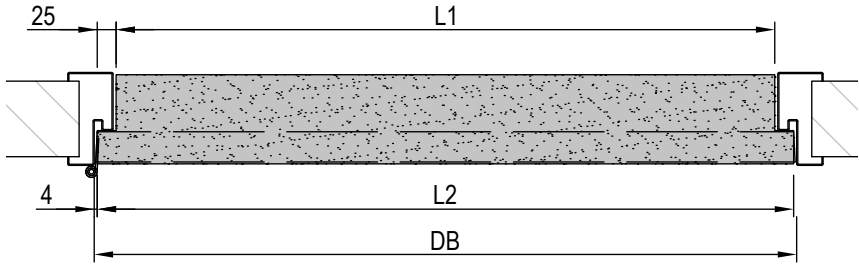
Bovenaanzicht stofdorpel
