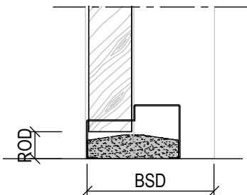
Stofdorpel met aangeschuinde oplooppvlak (1 of 2 zijdig) door aannemer te bepalen
