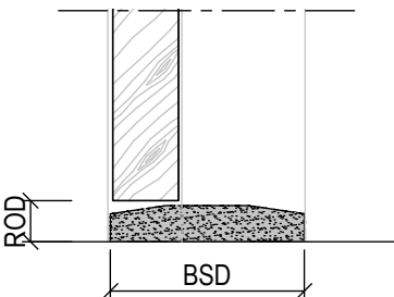
Stofdorpel met aangeschuinde oplooppvlak (1 of 2 zijdig) door aannemer te bepalen
