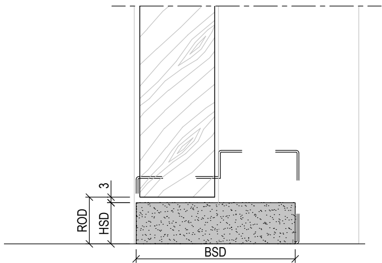
Stofdorpel recht
