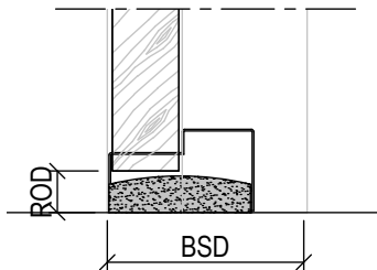
Stofdorpel met aangeschuinde oplooppvlak (1 of 2 zijdig) door aannemer te bepalen
