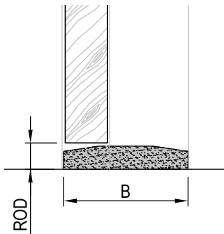
Stofdorpel met 1- of 2-zijdig aangeschuind oploophvlak, door aannemer te bepalen.
