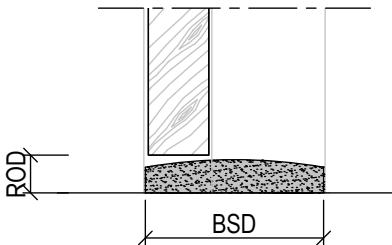
Stofdorpel met aangeschuinde oplooppvlak (1 of 2 zijdig) door aannemer te bepalen
