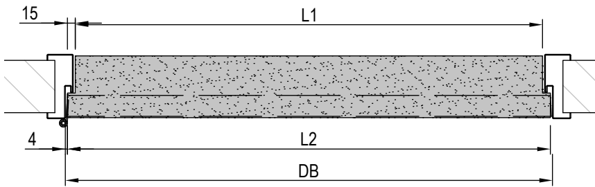
Bovenaanzicht stofdorpel
