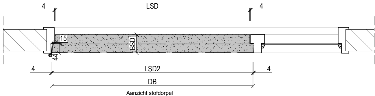
Aanzicht stofdorpel
