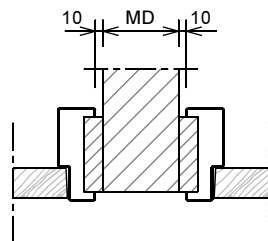
Aansluiting 2 kozijnen (losse afdekplaat optioneel leverbaar)
