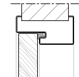
Optie: aanslagband 25 mm aanslagspinning
