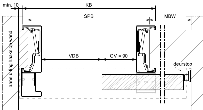
Horizontale doorsnede (aansluiting met metalstudwand)
