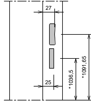
Slotgaten Nefef 4109
