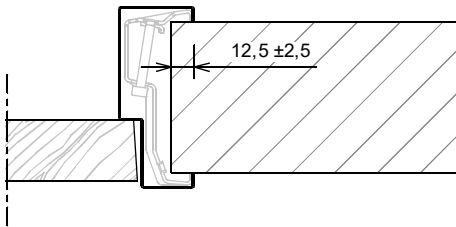
Aansluiting montagekozijn ( + klenbeugel )
