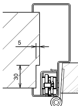
Uitkapping wand t.b.v. 3D scharnieropname
