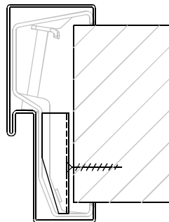
Wandbevestiging
