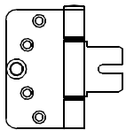
Scharnier A0838-IBW
