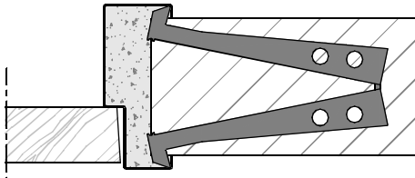
Aansluiting inmetSELkozijn ( + inleganker ) Optioneel: veiligheidsblokkers
