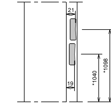
Slotgat Nemeff 1200 - 1300 - 1400 (woningbouw)
