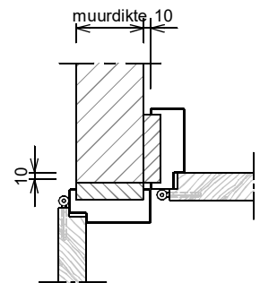
Hoekaansluiting 2 kozijnen
