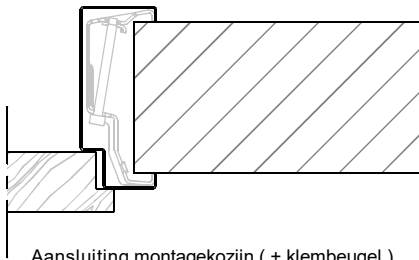
Aansluiting montagekozijn (+ klembeugel)
