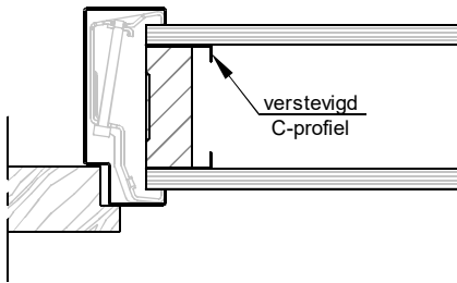
Aansluiting metalstudwand (+ klembeugel)
