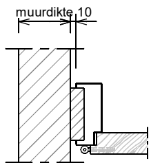
Aansluiting haakse wand
