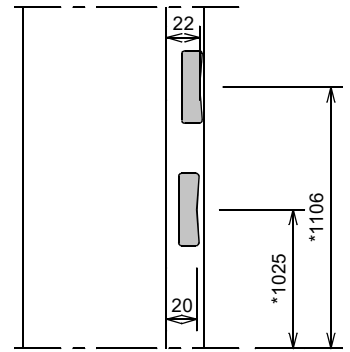
Slotgat Nemeff 600 (optioneel)
