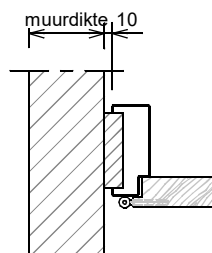
Aansluiting haakse wand
