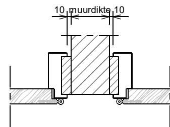
Aansluiting 2 kozijnen (losse afdekplaat optioneel leverbaar)
