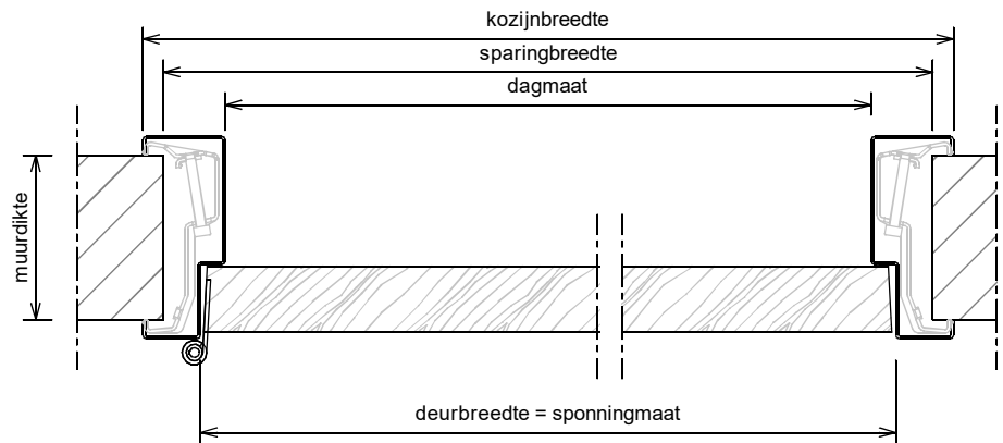
Horizontale doorsnede
