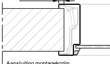
Aansluiting montagekozijn
