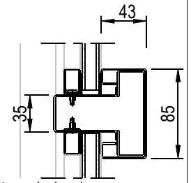
Borstwering met aanslagband spanning 15 mm
