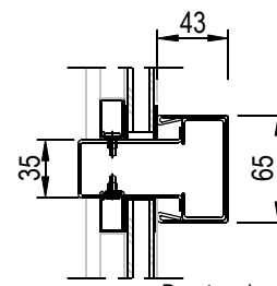
Borstwering met aanslagband spanning 15 mm
