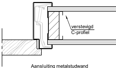
Aansluiting metalstudwand
