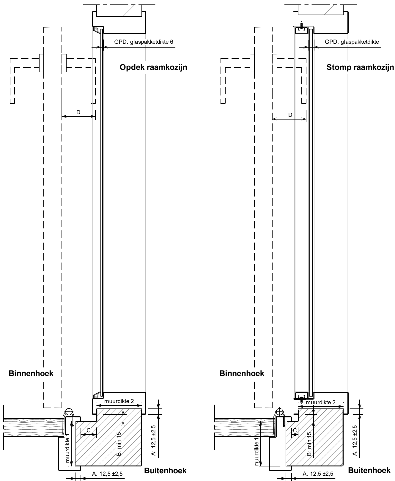
Buitenhoek 1 mm dik
