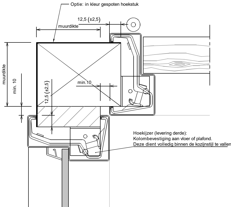
Hoekoplossing Kolom met aanslaglat
