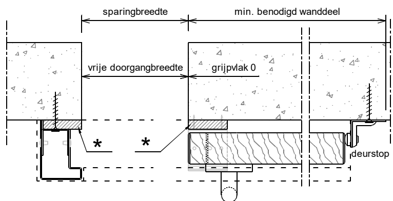
horizontale doorsnede grijpvlak 0
