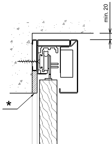
montage onder plafond
