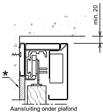
Aansluiting onder plafond
