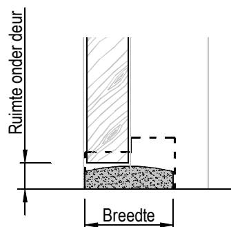
Stofdorpel gebold, door aannemer te bepalen.
