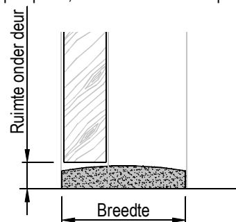
Stofdorpel met 1- of 2-zijdig aangeschuind oplooppvlak, door aannemer te bepalen.
