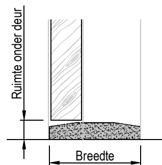
Stofdorpel met 1- of 2-zijdig aangeschuind opplovlak, door aannemer te bepalen.
