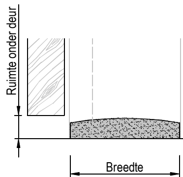
Stofdorpel gebold. Door aannemer te bepalen.
