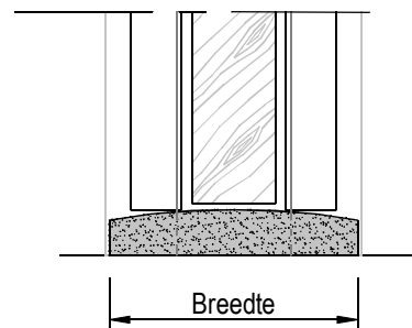
Stofdorpel gebold. Door aannemer te bepalen.
