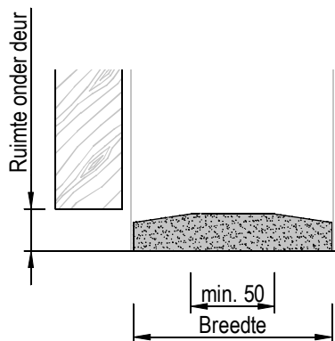
Stofdorpel met 1- of 2- zijdig aangeschuind oloopvlak. Door aannemer te bepalen.
