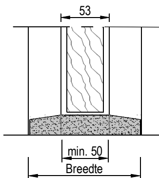
Stofdorpel met 1- of 2- zijdig aangeschuind oplooppvlak. Door aannemer te bepalen.
