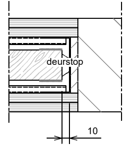
Grijpvlak 50 = deurstop 10
