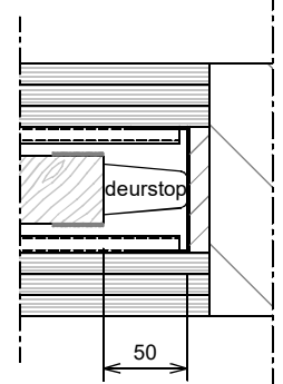
Grijpvlak 105 = deurstop 50
