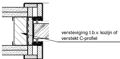
aansluiting MS-wand
