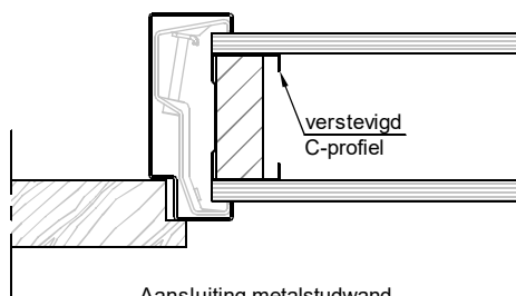
Aansluiting metalstudwand
