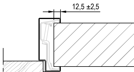
Aansluiting montagekozijn ( + klembeugel )
