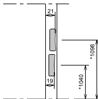
Slotgat Nemef 1200 - 1300 - 1400
