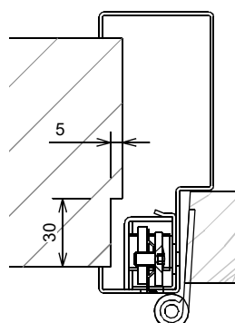
Uitkapping wand tbv 3D scharnieropname
