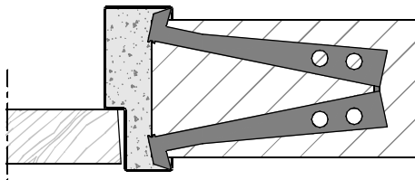
Aansluiting inmetsselkozijn ( + inleganker ) Optioneel: veiligheidsblokkers
