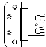
Scharnier Stiletto Inbraakwerend - Inmetssel-/ Montageuitvoering - sparringsmaten op aanvraag - max. 100 kg deurbladgewicht
