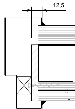
Dubbel gips Versterkingsplank (door derden)
