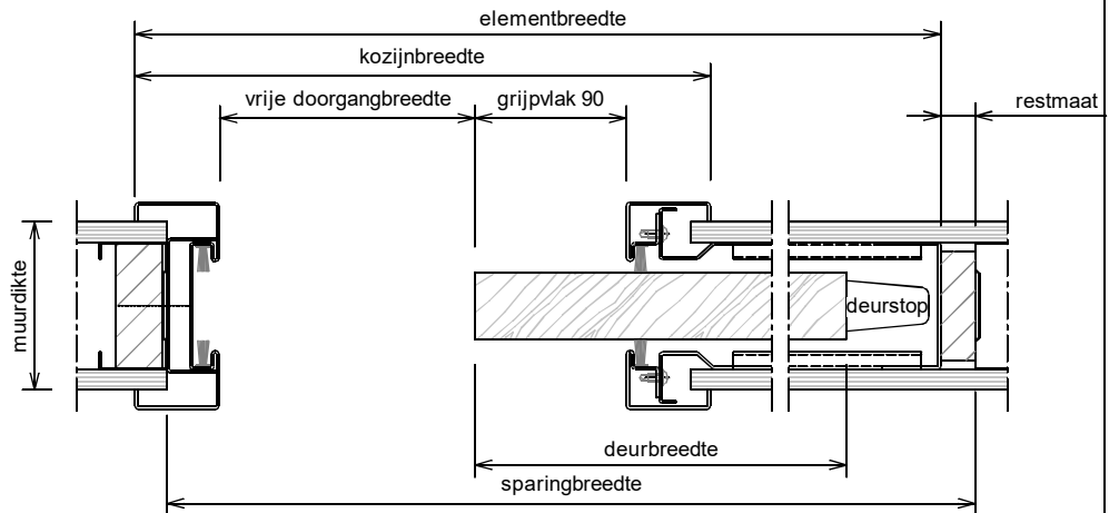
Horizontale doorsnede (aansluiting met metalstudwand)
