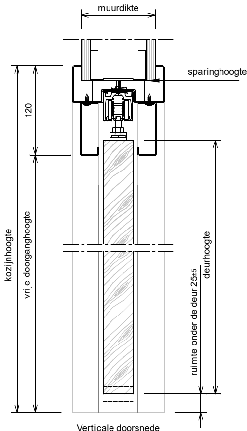
Verticale doorsnede
