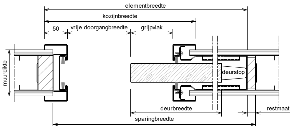
Horizontale doorsnede
