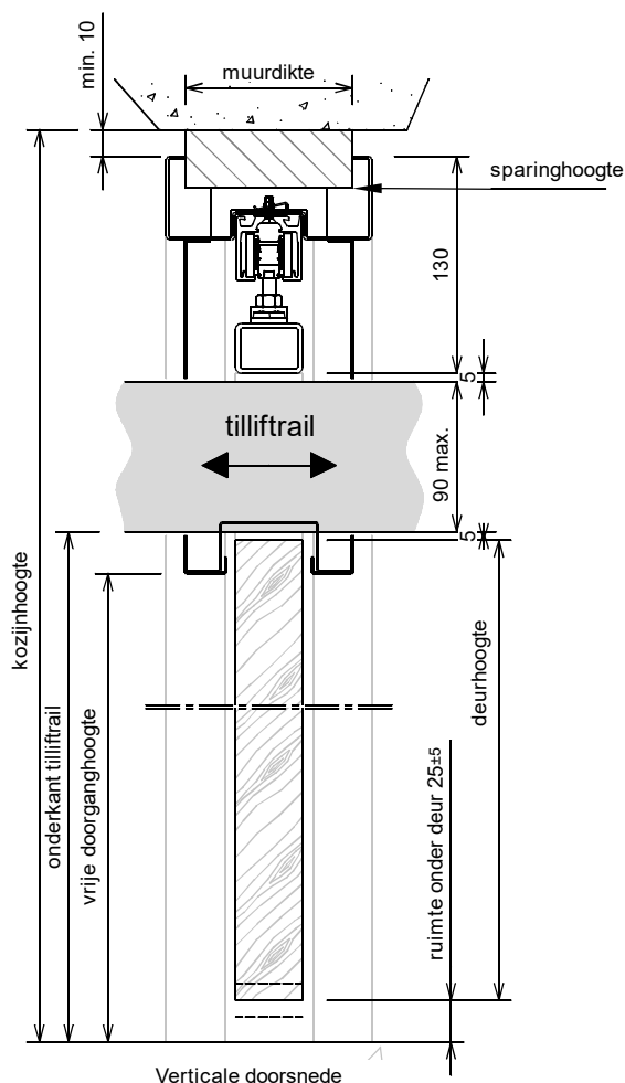
Verticale doorsnede
