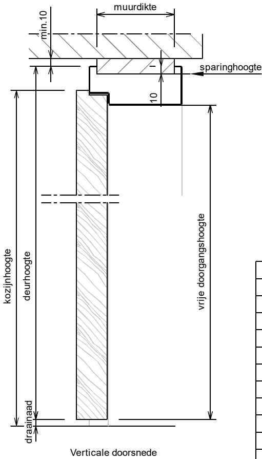
Verticale doorsnede
