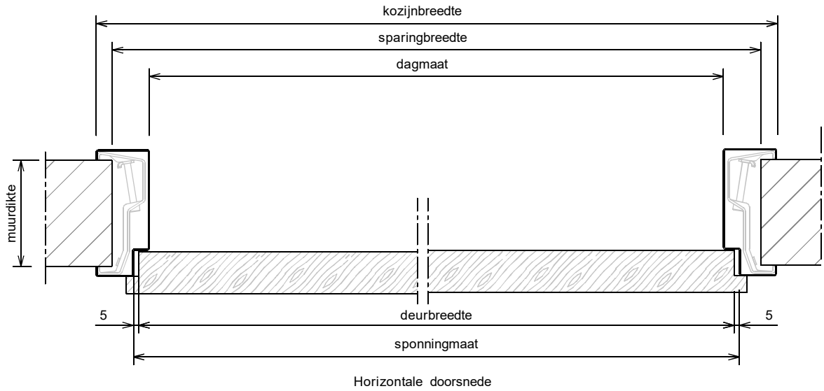
Horizontale doorsnede
