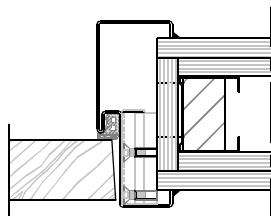
Stelblokje bij montage kozijn
