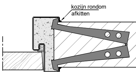
Optie: Aansluiting inmetselekozijn (kozijn compleet volgieten)
