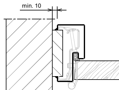
Aansluiting op haakse wand
