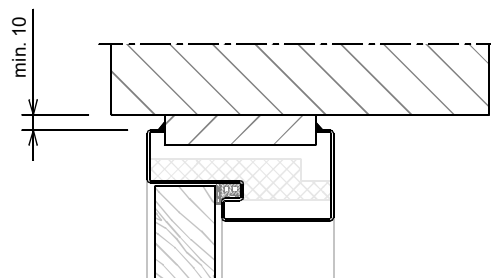
Aansluiting onder plafond
