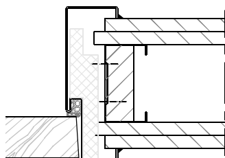
Optie: 15 mm aanslagsponning
