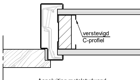
Aansluiting metalstudwand
