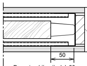
Deurstop bij grijpvlak 90
