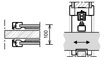
MD 100: per zijde 1x gipskartonplaat 12,5mm
