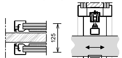
MD 125: per zijde 2x gipskartonplaat 12,5mm
