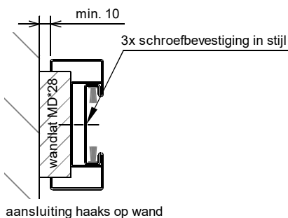
aansluiting haaks op wand
