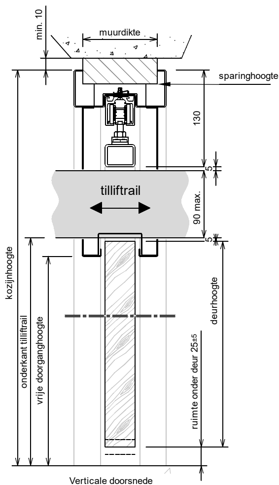
Verticale doorsnede
