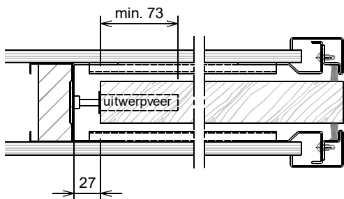
Deur volledig wegschuivend (grijpvlak 0) met uitwerpveer (optie)
