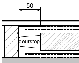
Deurstop bij grijpvlak 90
