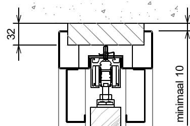
Aansluiting onder plafond
