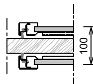
muurdikte 100: per zijde 1x gipskartonplaat 12,5mm
