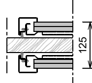
muurdikte 125: per zijde 2x gipskartonplaat 12,5mm
