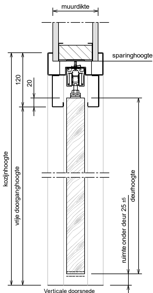
Verticale doorsnede
