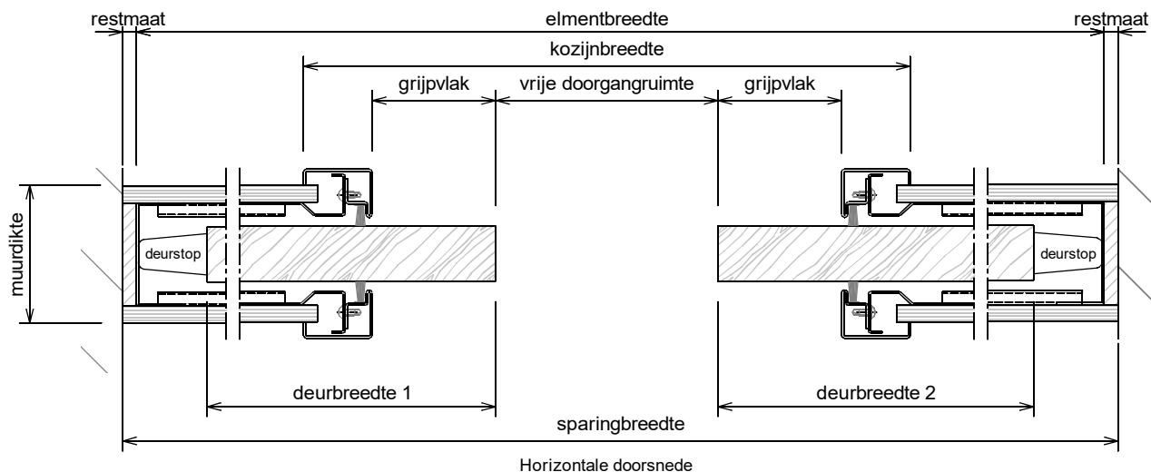
Horizontale doorsnede
