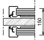
muurdikte 150: per zijde 3x gipskartonplaat 12,5mm
