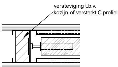
Aansluiting MS-wand
