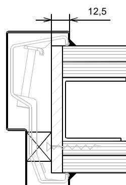
Optie: 2 of 3 gipsplaten: Verstevigingsplaat (door derden)
