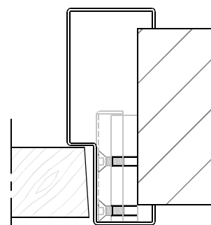
Stelblok (niet bij inmetSELkozijn)
