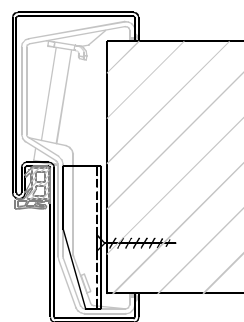
Wandbevestiging (niet bij inmetSELkozijn)
