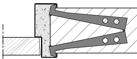
Aansluiting inmetSELkozijn ( + inleganker ) Optioneel: veiligingsblokkankers
