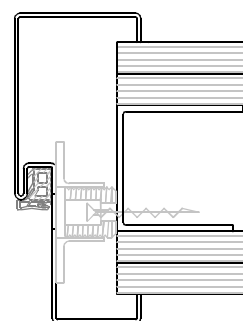
Borg- / Stelschotel (niet bij inmetSELkozijn)
